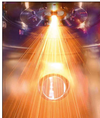
Atomizer z. Pulverschmelzedüse Verdüsung
