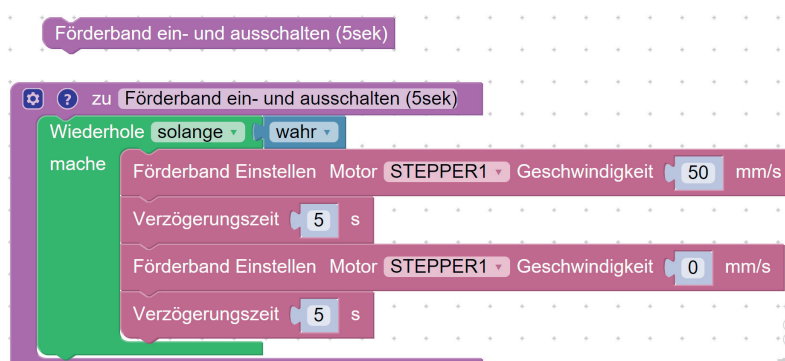
Abbildung 35: Lösung Übung 1b
