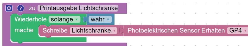
Abbildung 41: Definition der Lichtschranke als Variable (Auswahl des richtigen Ports beachten!)
