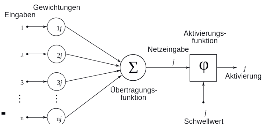
Abbildung 8: Darstellung eines Neuron-Modells 1
