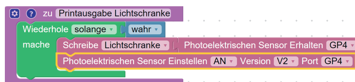
Abbildung 42: Einschalten der Lichtschranke
