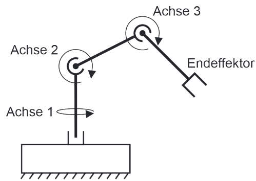
Abbildung 10: Schaubild 3-Achs-Kinematik
