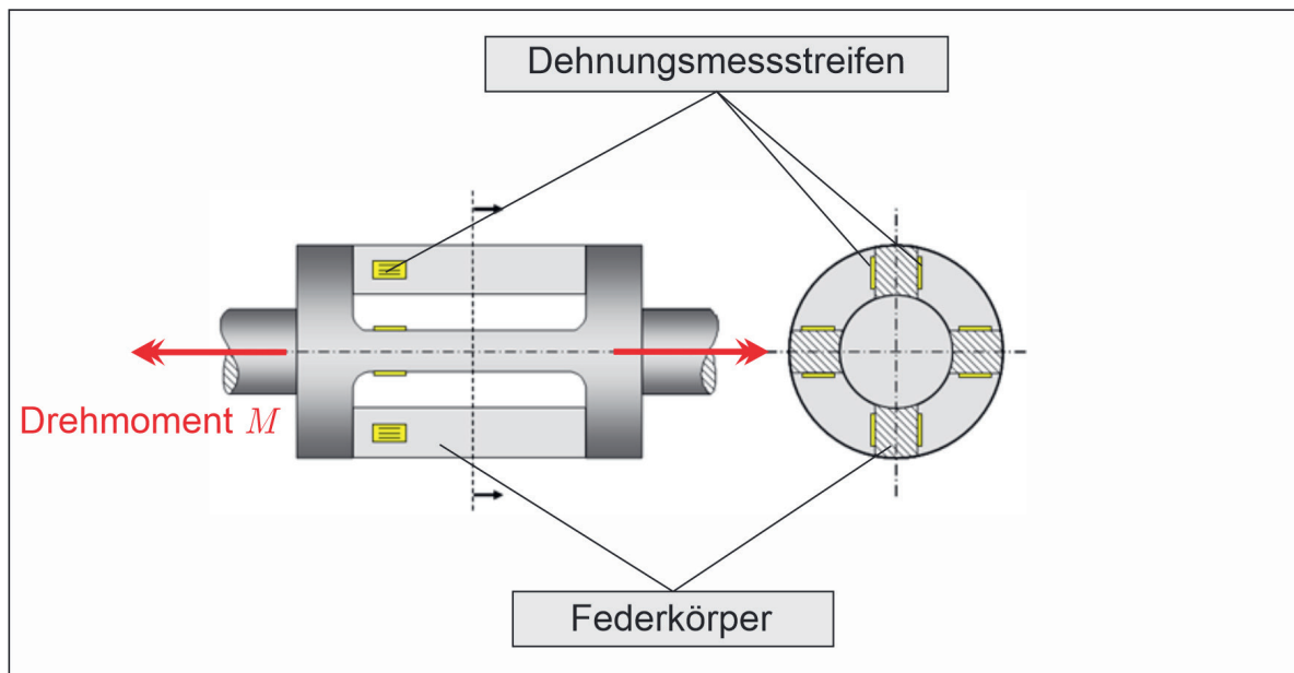
Abbildung 7: Drehmomentenaufnehmer [#Q5]
