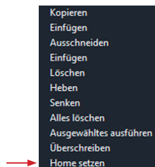
Abbildung 7: „Home setzen“
